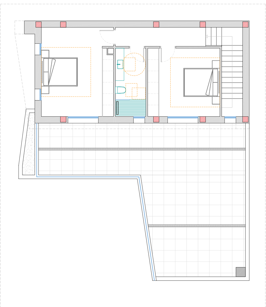
PLANTA PISO
