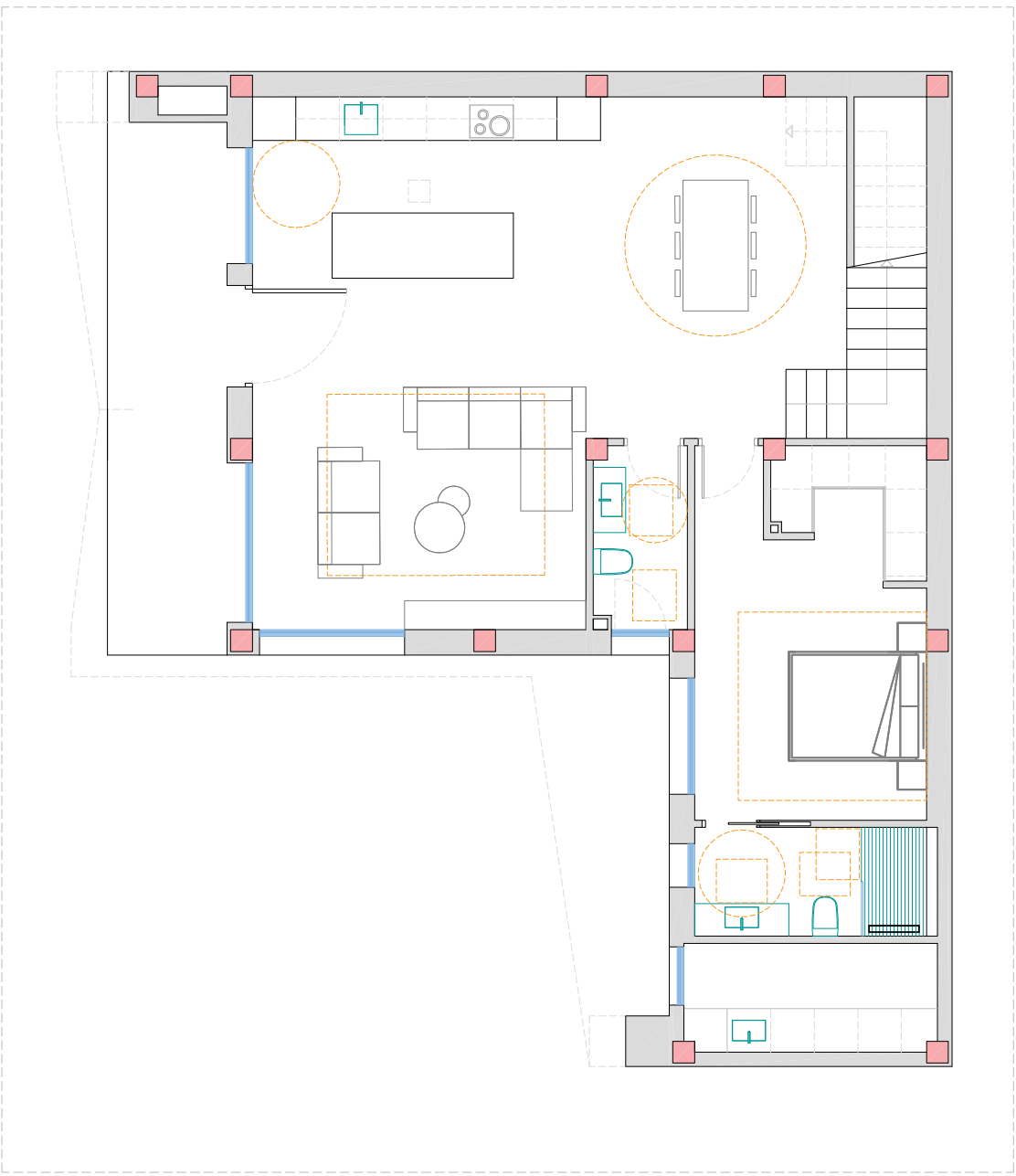
PLANTA BAJA
